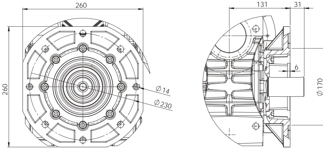
OPSİYONEL / OPTIONAL Çıkış Flanş / Output Flange
