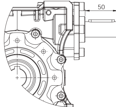
OPSİYONEL / OPTIONAL Pam Yeri Milli / Front Input Shaft
