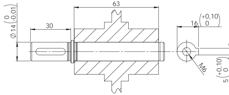
OPSİYONEL / OPTIONAL Tek Taraflı Çıkış Milli / Single Output Shaft
