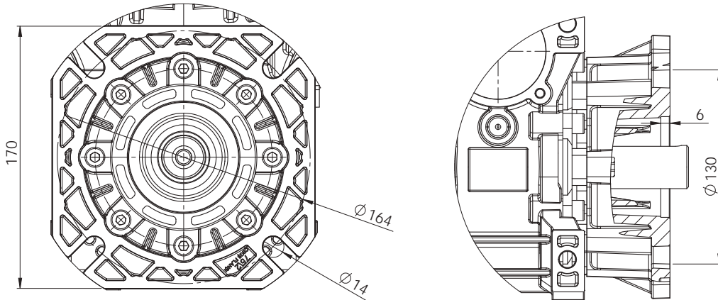
OPSİYONEL / OPTIONAL Çıkış Flanşı / Output Flange
