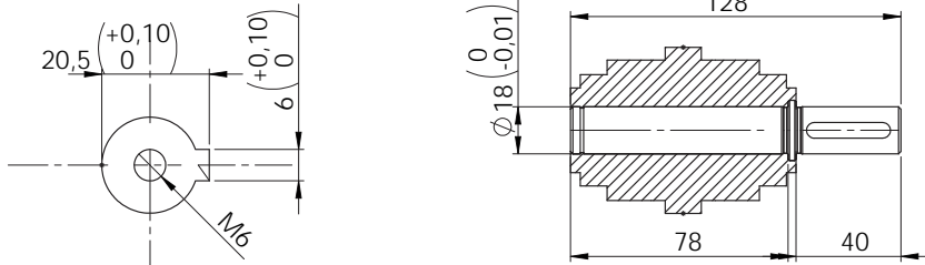
OPSİYONEL / OPTIONAL Tek Taraflı Çıkış Millı / Single Output Shaft
